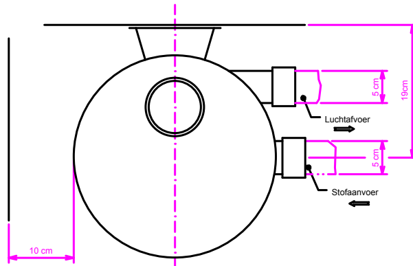
Bovenaanzicht MK 18 stofzuigunit
